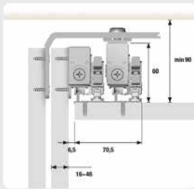
Άνω ράουλο για εξωτερικό φύλλο πόρτας
