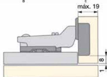
Μεντεσές για 19άρα πόρτα
