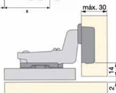
Μεντεσές για 30άρα πόρτα
