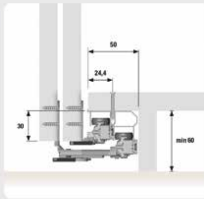
Άνω ράουλο για εσωτερικό φύλλο πόρτας
